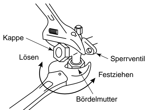
Ventil SP56 gasseitig
