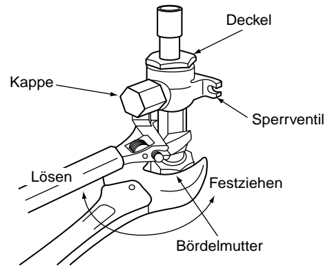
Ventil SP80 gasseitig
