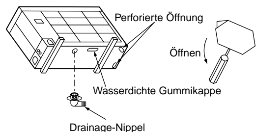
Wasserdichte Gummikappe
