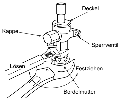
Ventil auf Gasseite
