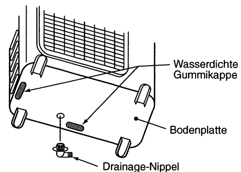
Drainage-Nippel
